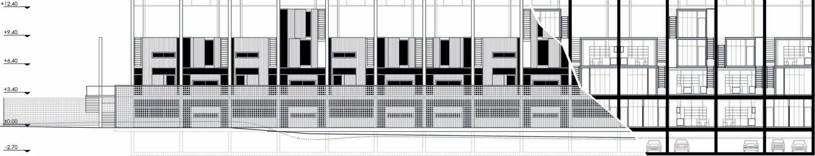
ΝΟΤΙΑ ΟΨΗ \ ΔΙΑΜΗΚΗΣ ΤΟΜΗ ΣΥΓΚΡΟΤΗΜΑΤΟΣ Α | ΚΛΙΜΑΚΑ 1:200
