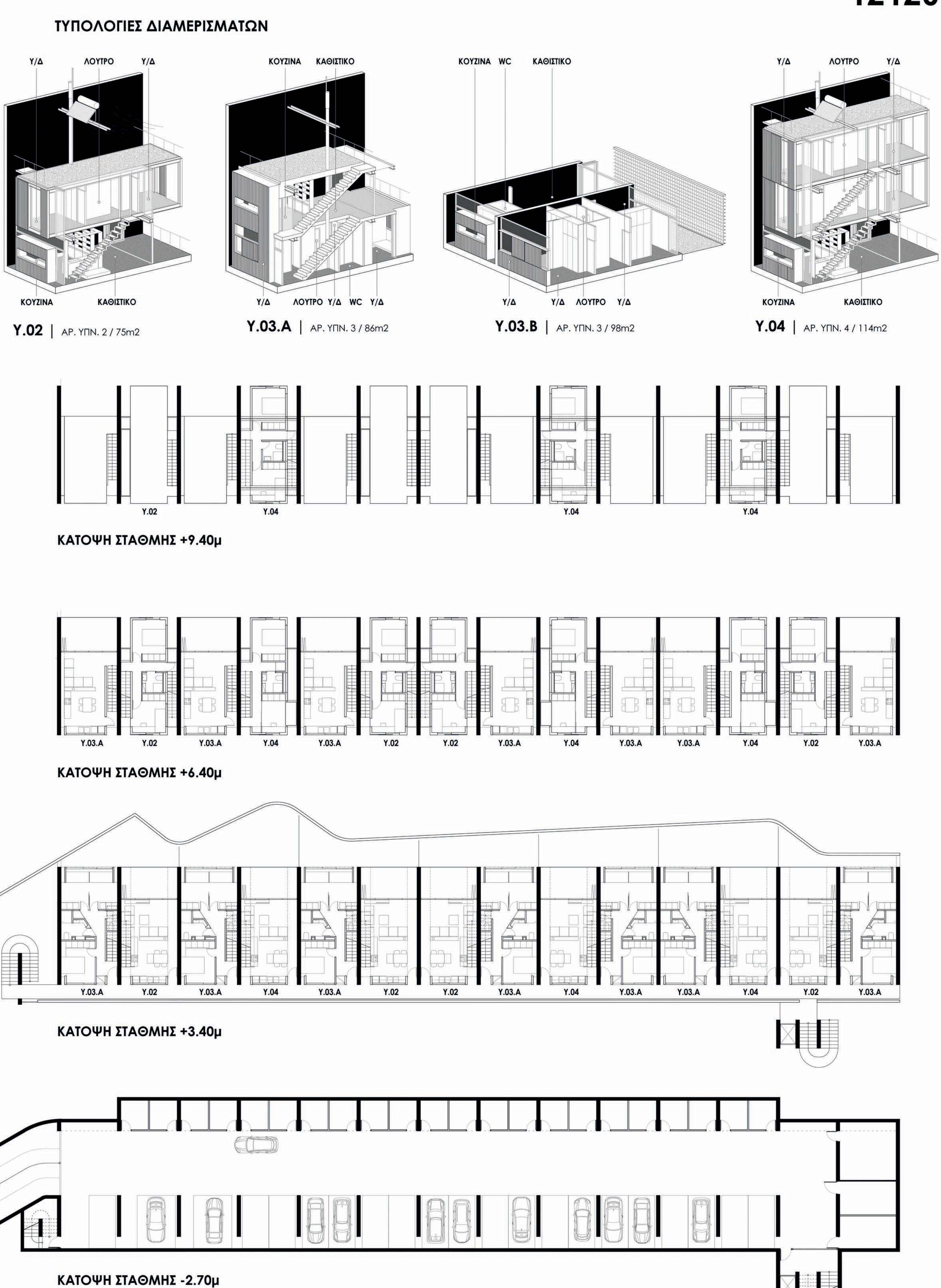
ΣΥΓΚΡΟΤΗΜΑ Α | ΑΡ. ΔΙΑΜΕΡΙΣΜΑΤΩΝ: 21 | ΚΛΙΜΑΚΑ 1:200
