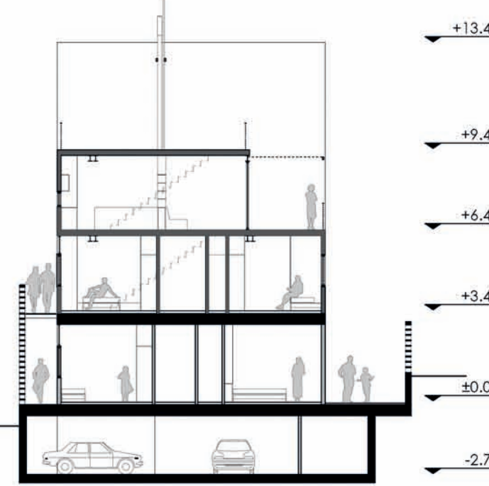
ΤΟΜΗ Γ | ΚΛΙΜΑΚΑ 1:200
