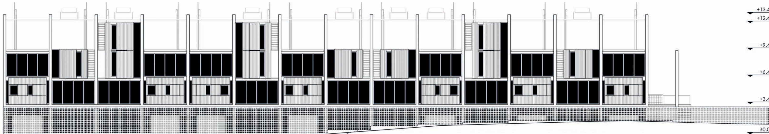
ΒΟΡΕΙΑ ΟΨΗ ΣΥΓΚΡΟΤΗΜΑΤΟΣ Α | ΚΛΙΜΑΚΑ 1:200
