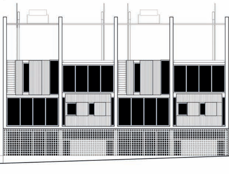
ΑΝΑΤΟΛΙΚΗ ΟΨΗ ΣΥΓΚΡΟΤΗΜΑΤΟΣ Β | ΚΛΙΜΑΚΑ 1:200
