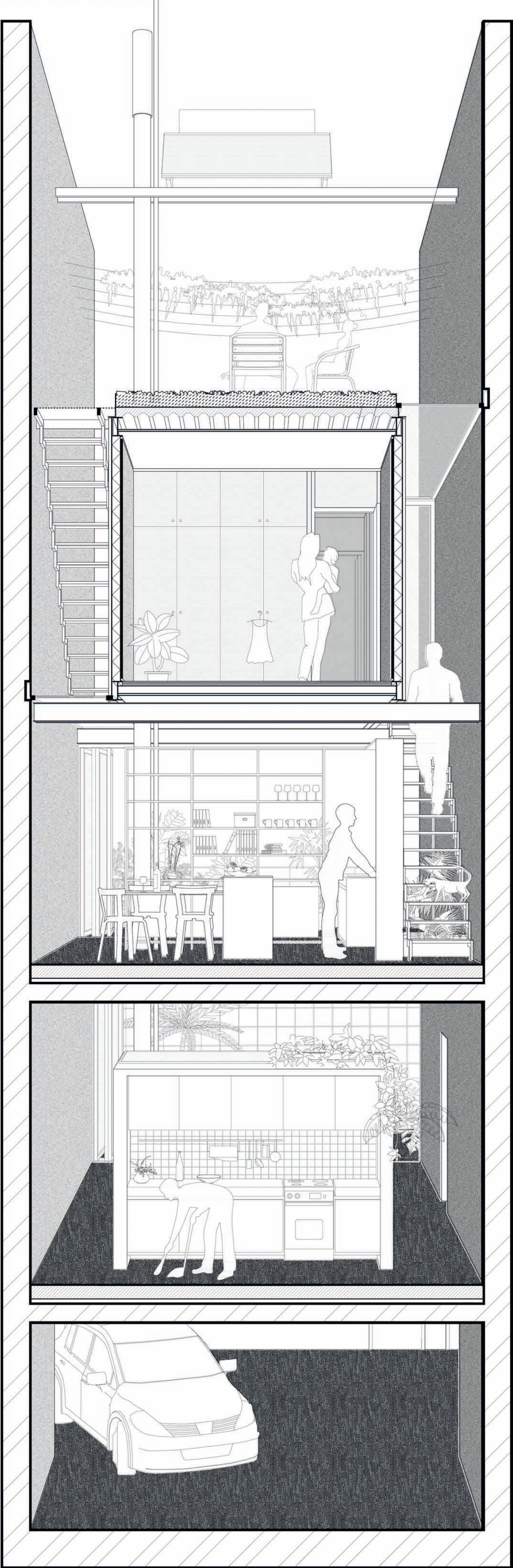
ΕΓΚΑΡΣΙΑ ΠΡΟΟΠΤΙΚΗ ΤΟΜΗ ΜΟΝΑΔΑΣ
